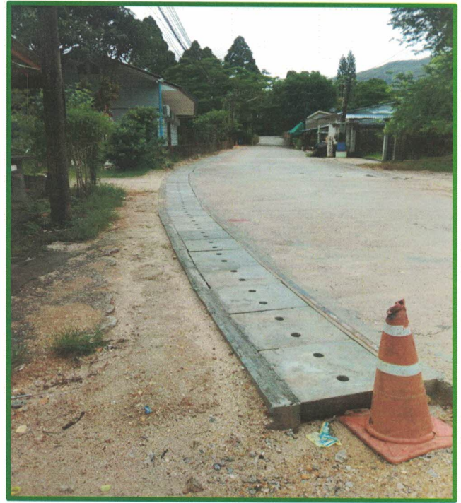
18. โครงการก่อสร้างรางระบายน้ำ ค.ส.ล. รูปตัวยู ซอยประชาพิทักษ์ (ซอยข้างโรงพัก)
